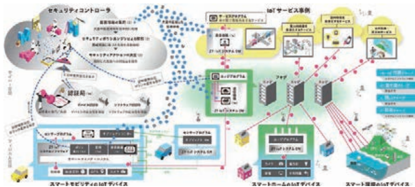
図：ゼロトラストIoTシステムの概要
