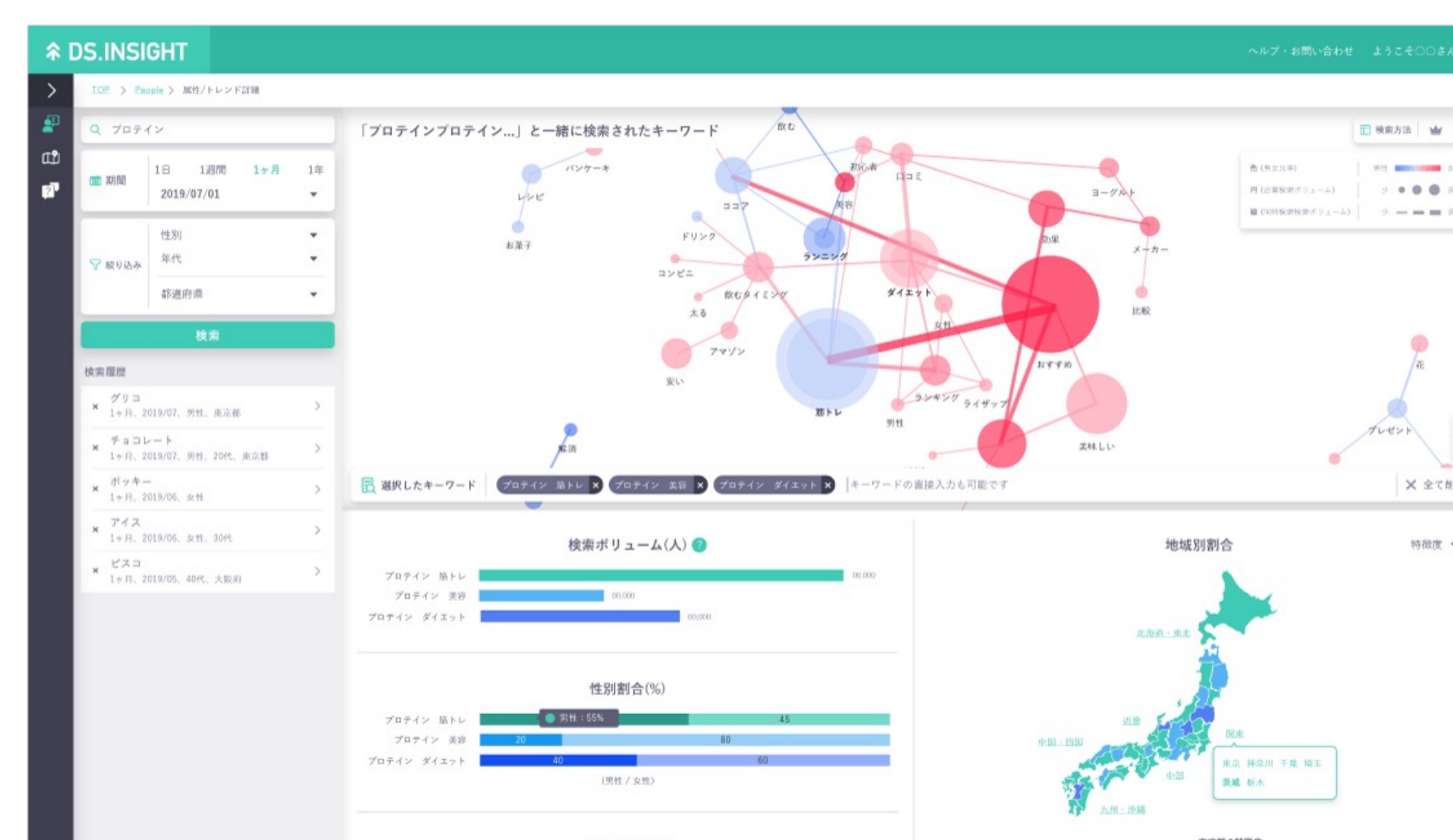
DS.INSIGHT(WEB検索)
